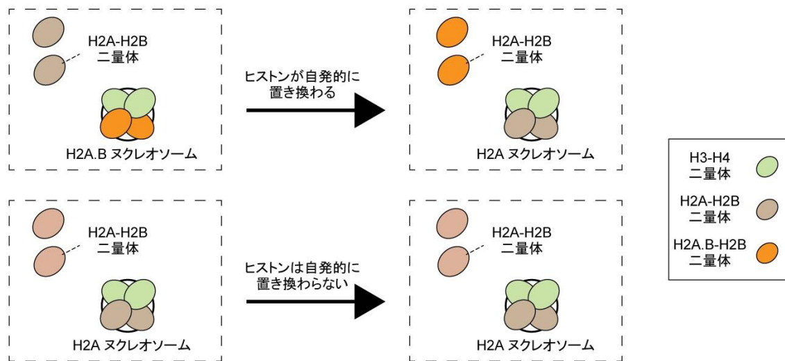
図 2. H2A.B ナクレオソームの自発的に ヒストン が置き換わる 性質 H2A.B ナクレオソーム中の H2A.B-H2B 二量体が、溶液中に存在する主要型の H2A-H2B 二量体と自発的に置き換わ るという、新規の動態を発見しました。
