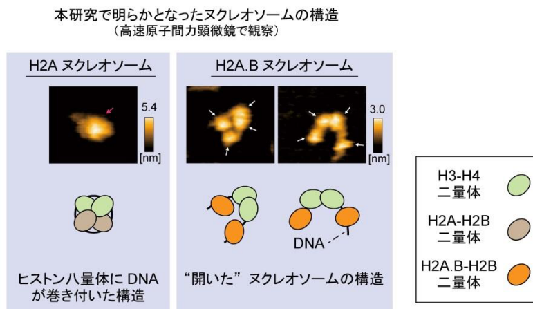
図 3. H2A.B ナクレオソーム を高速原子間力顕微鏡で観察した像 高速原子間力顕微鏡による解析から、H2A.B ナクレオソームは、主要型ヒストンでは見られないナクレオソームが“開いた”構造を取る ことが明らかとなりました。赤および白矢印は、それぞれヒストン八量体および二量体と考えられるものを指しています。高速原子間力顕微鏡像の下に模式図を示しています。
